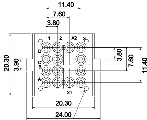
MATING RELAY STOP POST PLOTS D'APPUI DU RELAIS
